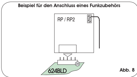
Beispiel für den Anschluss eines Funkzubehörs
